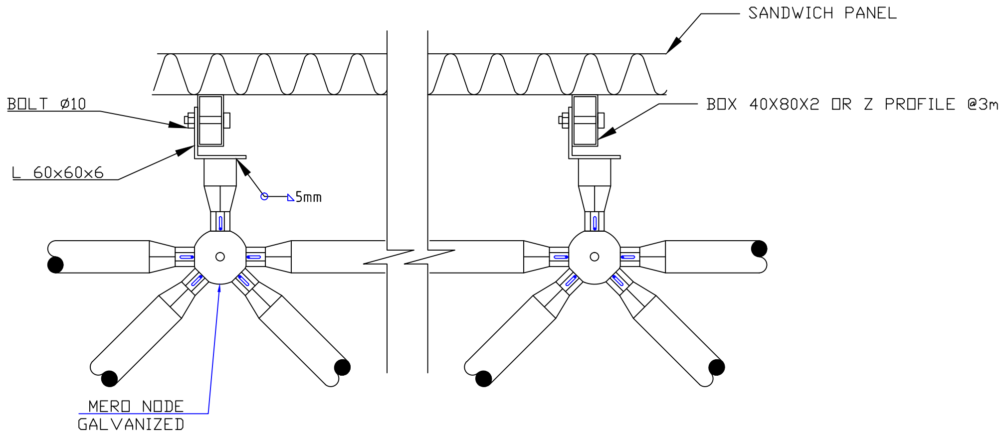
جزئیات اتصال پوشش به سازه
